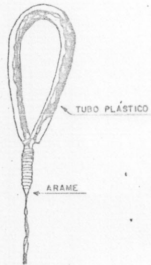
DET.II.b) - PROTEÇÃO DA ALÇA DO ESTOPRO
